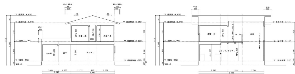
断面図
