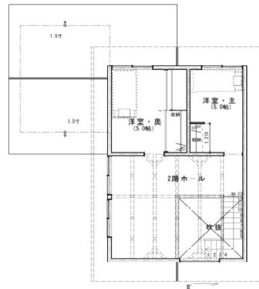
2F 平面図
