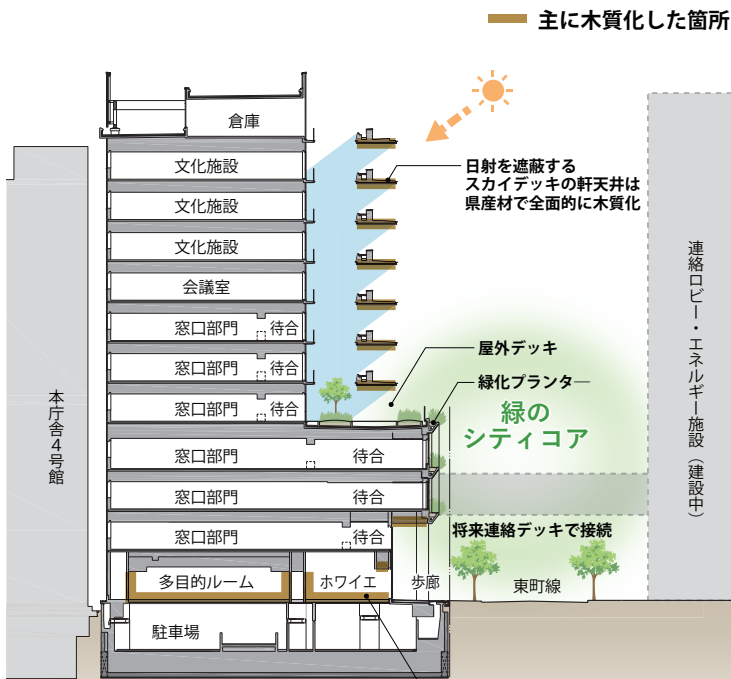
■ スカイデッキによる彫りの深い東面ファサード。街路に面した街並みの一部として、夜間は間接的な光で照らし、神戸市の新たな夜間景観を象徴する
